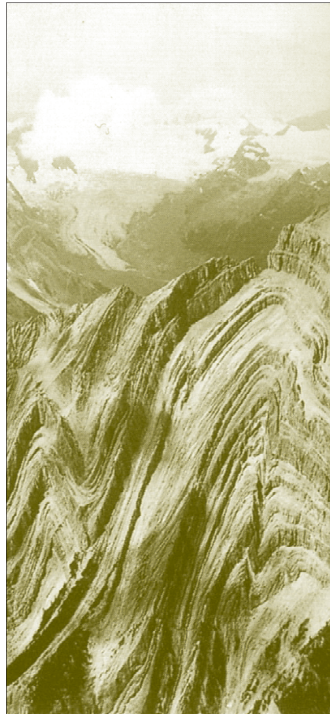
„Gefaltene Gebirge“ aus H.-H. Zillmer, Darwins Irrtum , Abb. 81.
